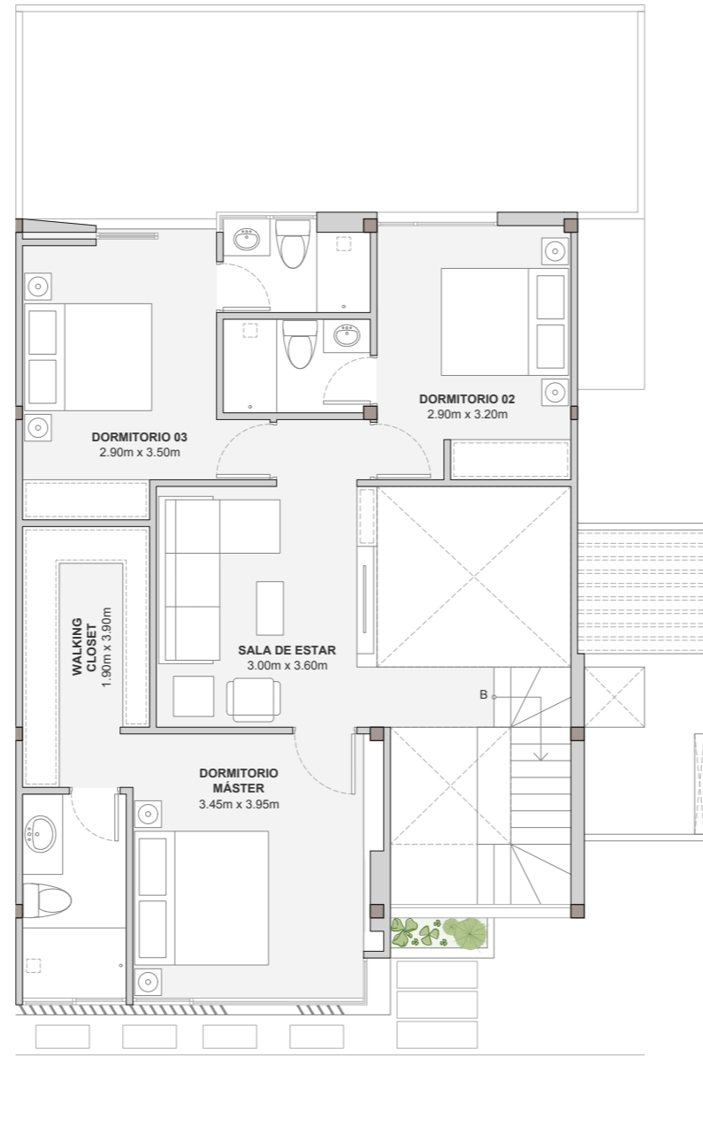
PLANTA ALTA
