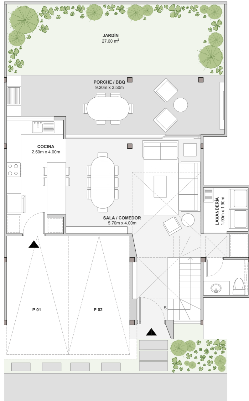
PLANTA BAJA
